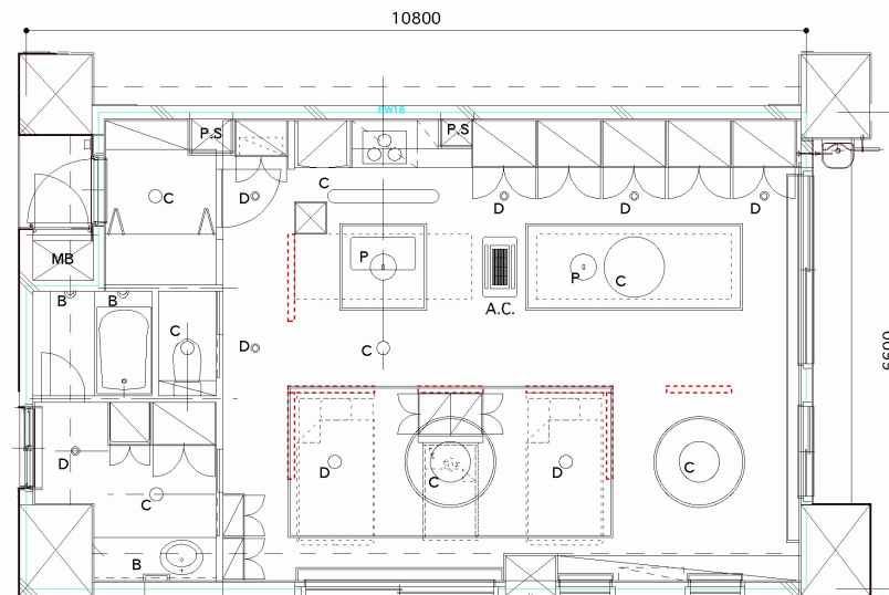
住戸天井伏図
